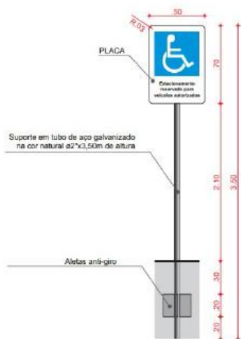
Sinalização vertical vaga PCR
